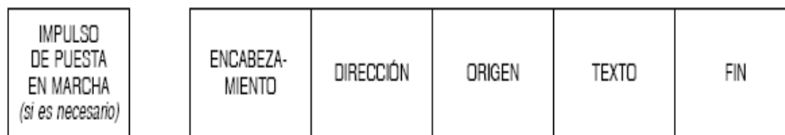
Figura 4-2. Forma de transmisión — operaciones de teleimpresor (véase 4.4.10.1.2)
